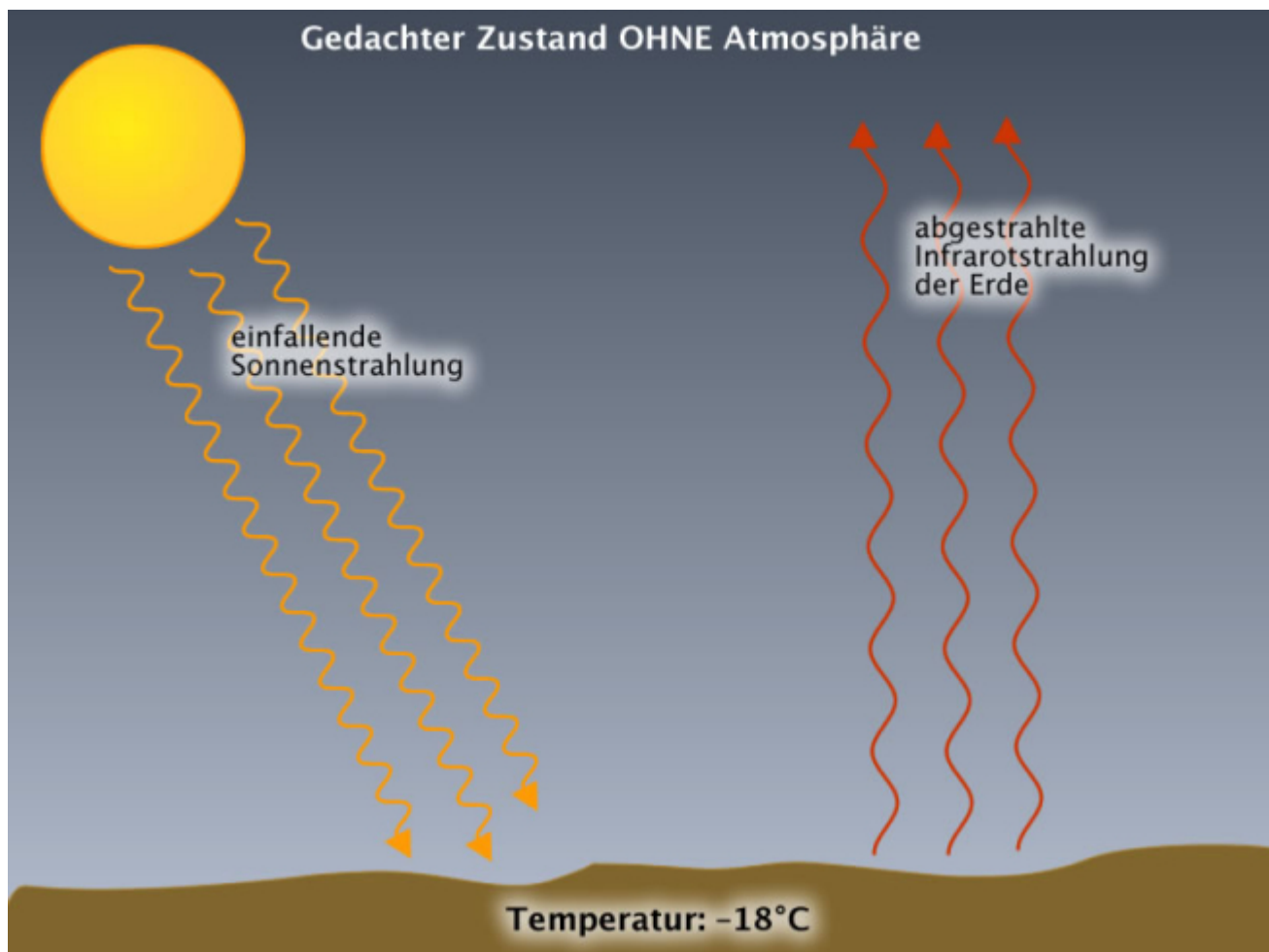
Abb. 2: Gedankenexperiment: Vereinfachter Strahlungshaushalt der Erde ohne Atmosphäre. Quelle:
