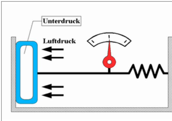
Abb. 3: Funktionsprinzip eines Dosenbarometers
